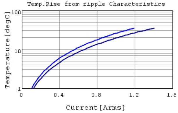
GRM155R61C224KA12 Temp.rise — 600kHz —
