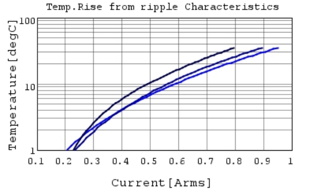
GRM1555C1H100JA01 Temp.rise 700MHz
