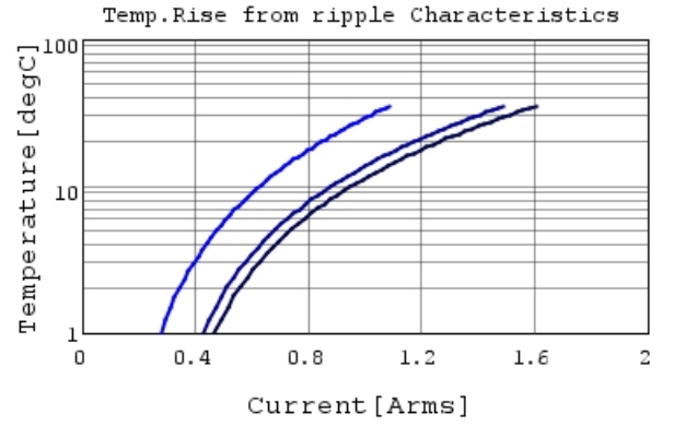
GCM188R71C104KA37 Temp.rise — 400kHz
