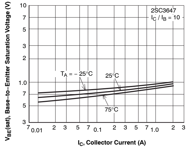
Figure 15. V_{BE}(sat) - I_C
