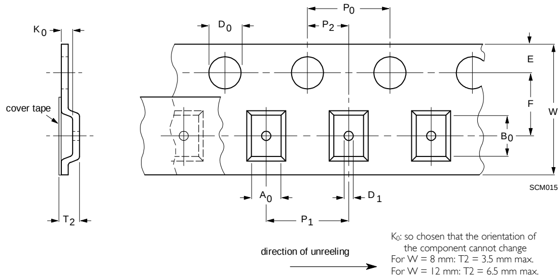
Fig. 4 Blister tape
