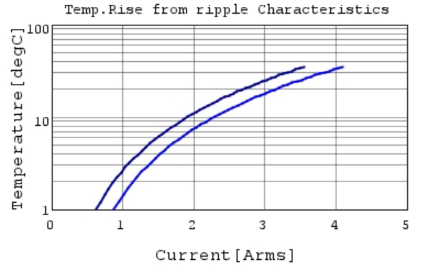
GRT21BR71H105KE01 Temp.rise — 500kHz —
